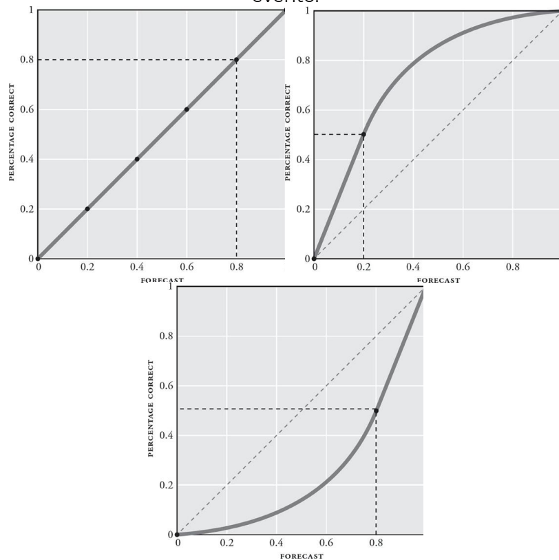
Figura 1 – Exemplos de calibração perfeita, underconfident e overconfident quando comparada a probabilidade de ocorrência prevista e a porcentagem correta do evento.
