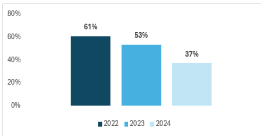
Gráfico 5 - Projeção PCA 2024
